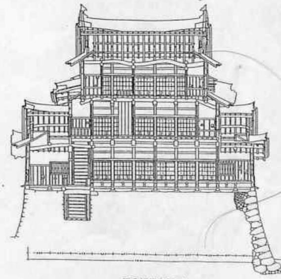
天守桁行断面図
